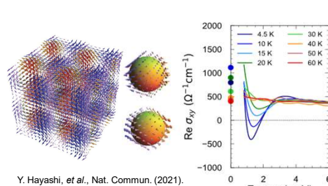
(3次元) スキルミオンによる異常・トポロジカルホール共鳴
