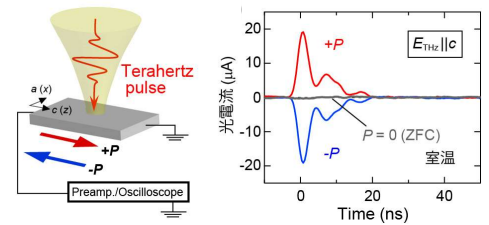
ソフトフォノン励起による光起電力効果
