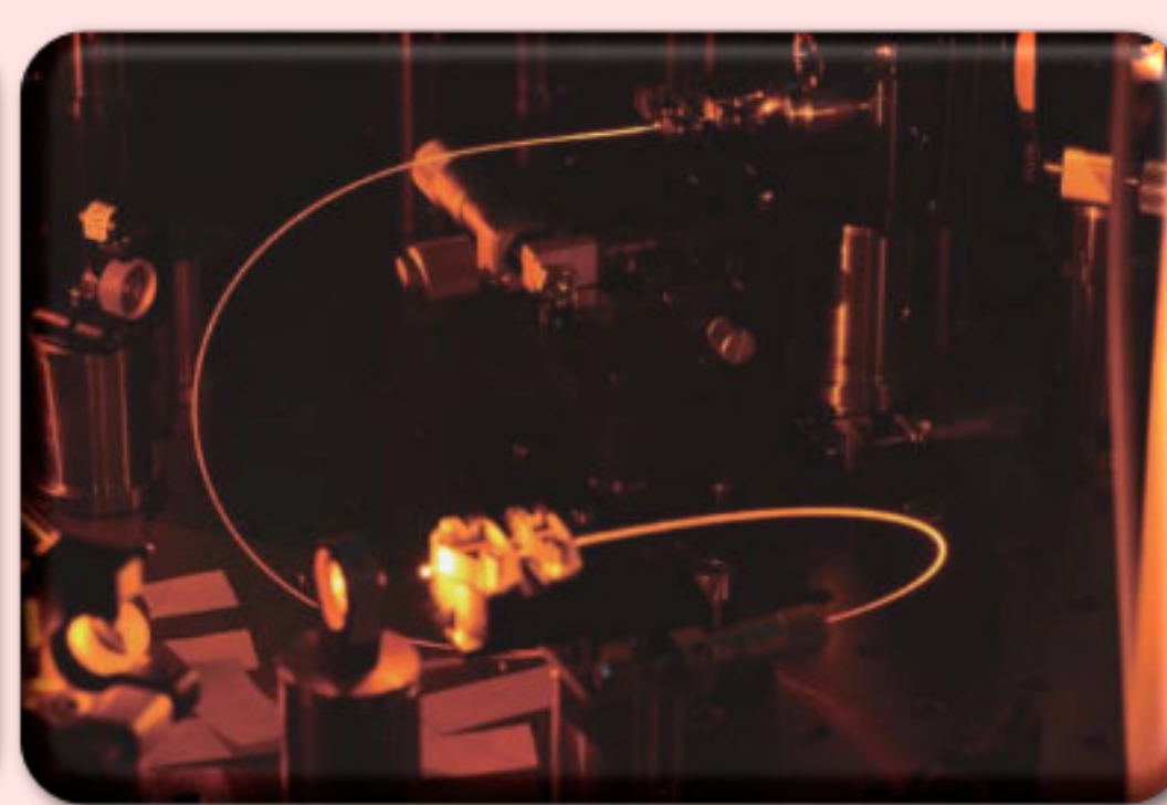
世界最大級の30 mフェムト秒外部共振器
