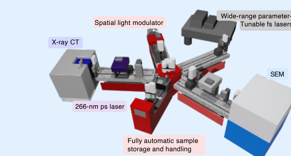
全自動レーザー加工データ収集システム
